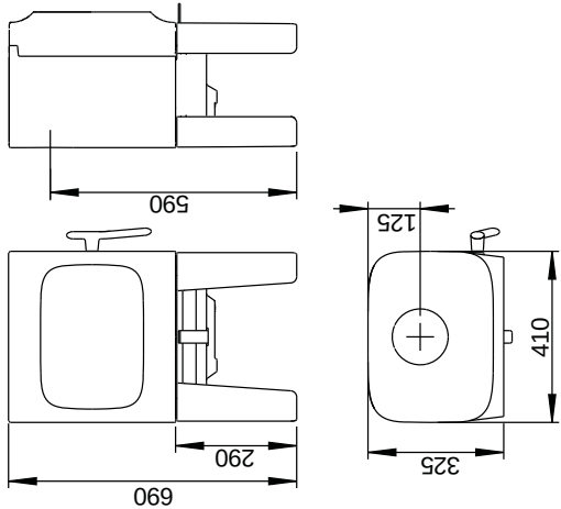
Jøtul F 105 R lange ben
