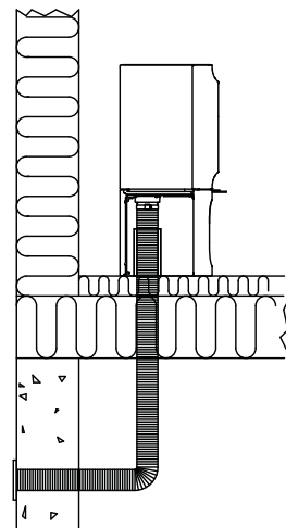
Figur 2C, gjennom golv og kjeller
