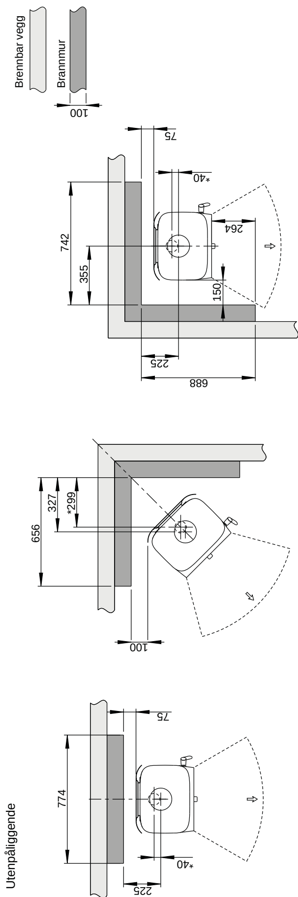
Jøtul F 105 Min. avstand til brennbar vegg beskyttet av brannmur
